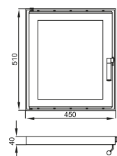
Drzwiczki piecove bezramowe szyba duplex
